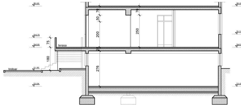
PRESEK 1-1 - POSTOJEĆE STANJE
