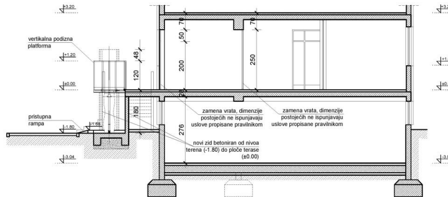
PRESEK 1-1 - NOVOPROJEKTOVANO STANJE
