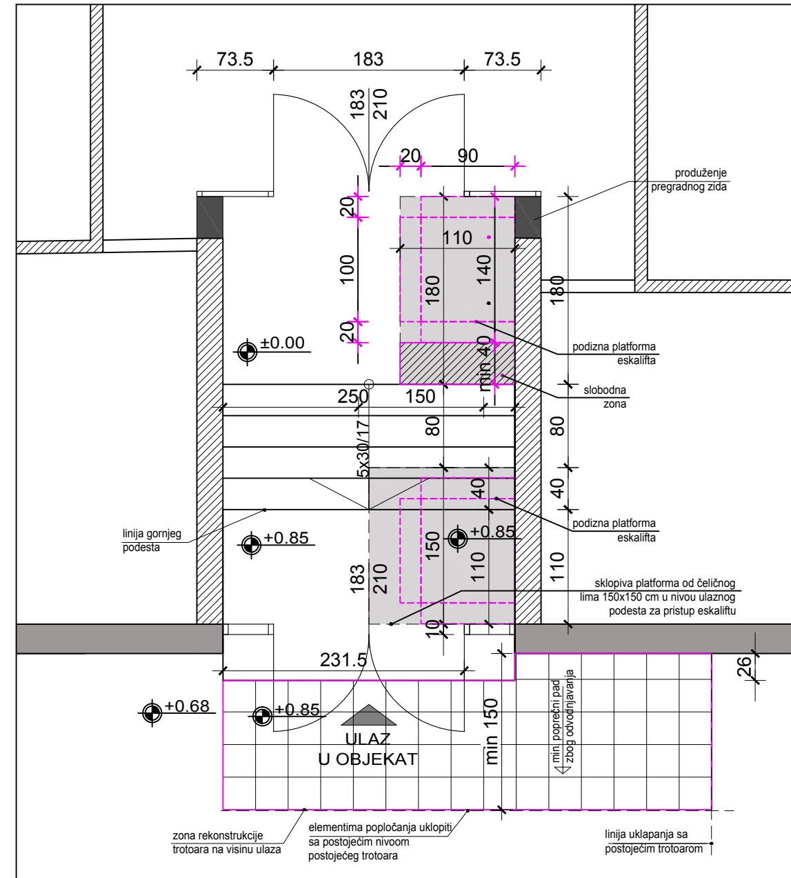
B NOVOPROJEKTOVANO STANJE - OSNOVA ULAZNOG VETROBRANA SA OTVORENOM PODIZNOM PLATFORMOM
