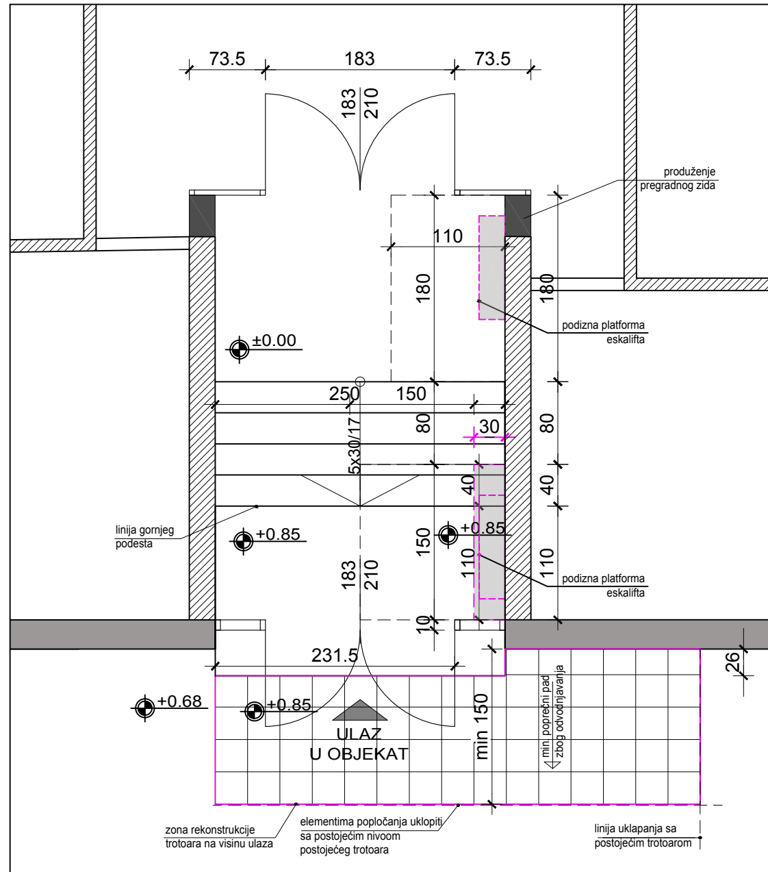
A NOVOPROJEKTOVANO STANJE - OSNOVA ULAZNOG VETROBRANA SA SKLOPLJENOM PODIZNOM PLATFORMOM
