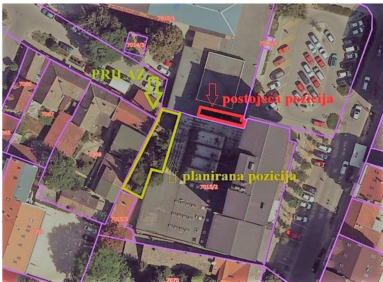
Приказ измештања протипожарног ступеништа
